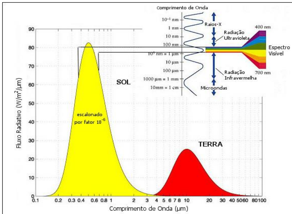
Figura 10 - Intensidade da radiação emitida versus o comprimento de onda para um corpo negro ideal. Fonte: http://recursosolar.geodesign.com.br/Pages/Sol_Rad_Basic_RS.html . Acesso: 15/04/2021.
