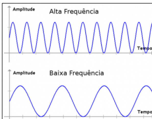
Figura 3 – Representação esquemática de duas ondas com frequência diferentes. Na onda superior, a onda tem frequência alta, enquanto na inferior a onda tem frequência baixa.
