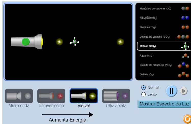
Figura 16: Interação da luz visível com a molécula de metano. Fonte: autora.
