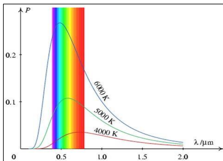
Figura 9 - Intensidade da radiação emitida versus o comprimento de onda para um corpo negro ideal. Fonte: http://portaldoprofessor.mec.gov.br/fichaTecnicaAula.html?aula=23505 . Acesso: 10/12/2020.
