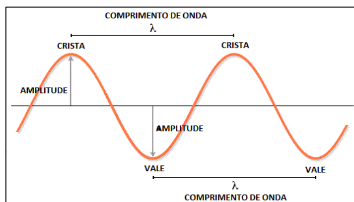
Figura 2 – Representação esquemática do conceito de comprimento de onda e da amplitude da onda. Fonte: https://athoselectronics.com/frequencia-como-funciona/ . Acesso: 10/12/2020.
