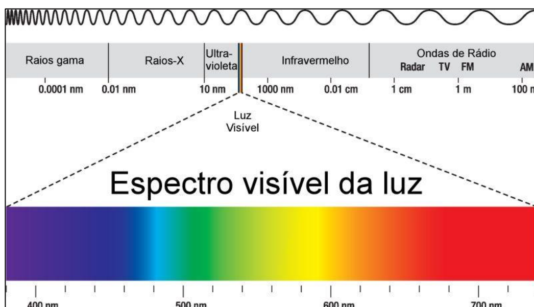
Figura 5 - Espectro eletromagnético. Fonte: https://www.todamateria.com.br/espectro-eletromagnetico/ . Acesso: 10/12/2020
