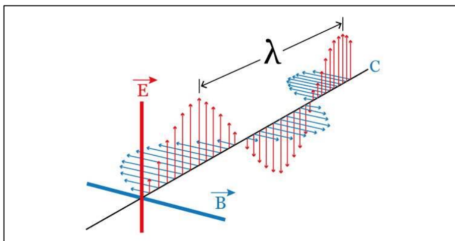
Figura 4 - Propagação da onda eletromagnética. Fonte:
