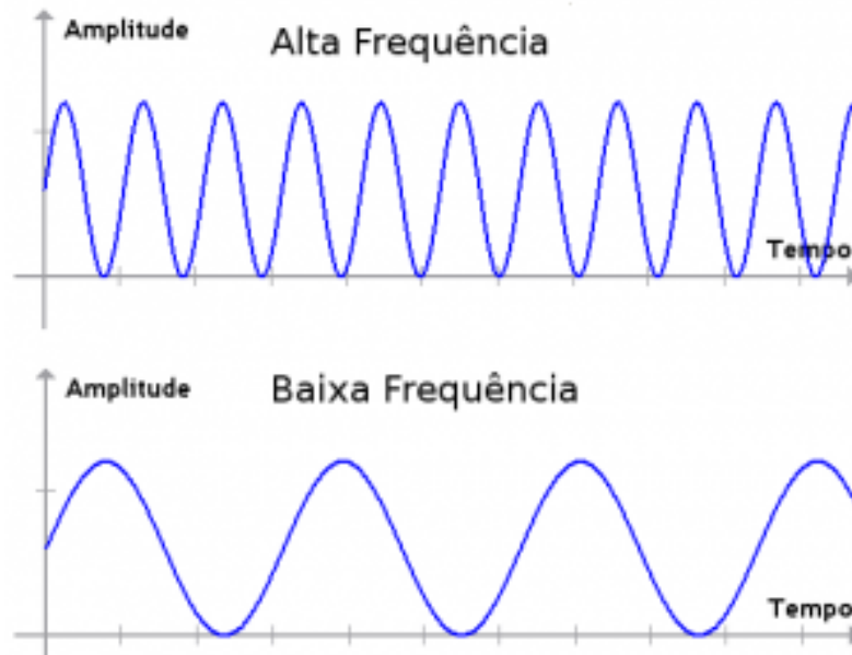
Figura 4: Frequência da onda. Fonte: https://magroove.com/blog/pt-br/frequencia/ . Acesso: 03/08/2020.
