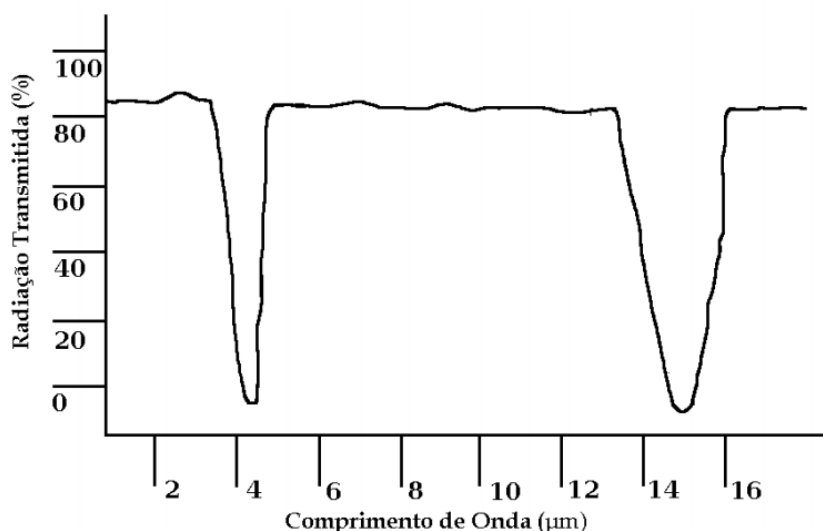
Figura 11 - Espectro do infravermelho da molécula de \text{CO}_2 . Fonte: Junges et al., 2018.
