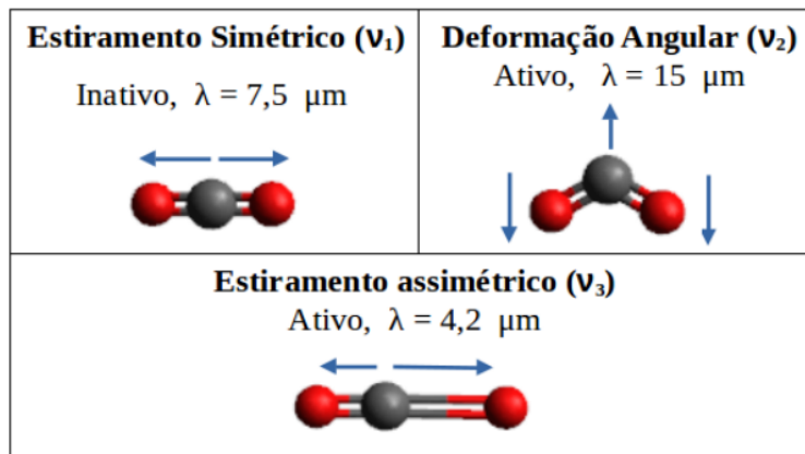
Figura 12 - Os modos normais de vibração do \text{CO}_2 . Fonte: Junges et al., 2018.
