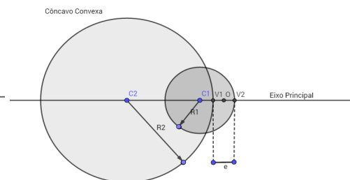
Figura 3: Lente Côncavo Convexa
