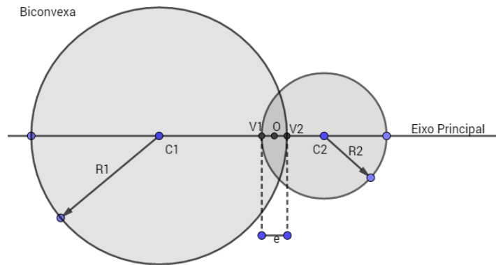
Figura 14 - Raio de curvatura e centro óptico de uma lente biconvexa.
