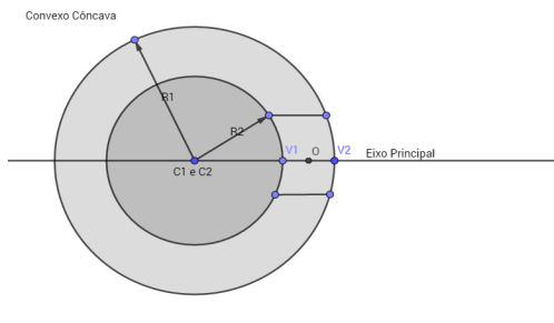
Figura 7: Lente Convexo Côncava
