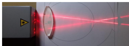
Figura 4: Laser e lente biconvexa
