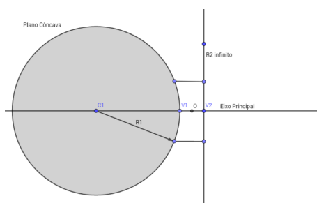
Figura 6: Lente Plano Côncava
