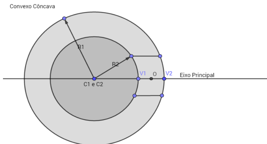
Figura 20: Lente convexo côncava com a identificação de cada componente óptico.
