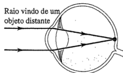
Figura 40 - Olho normal
