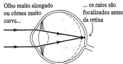
Figura 30 - Olho míope
