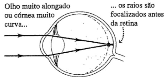
Figura 41 - Olho míope
