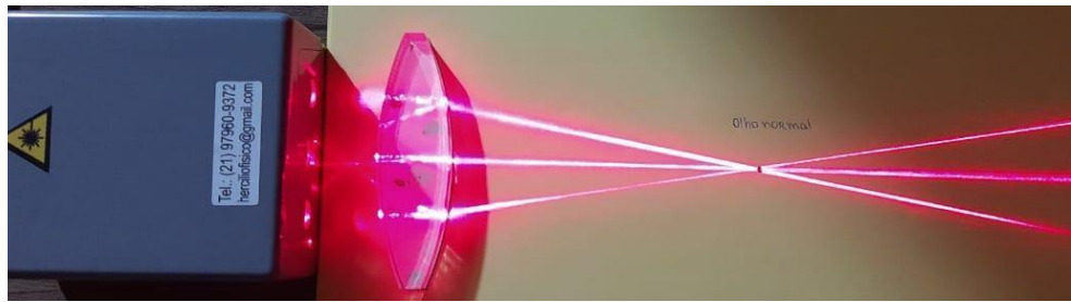
Figura 47: Olho normal
