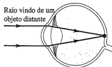
Figura 22 - Olho normal
