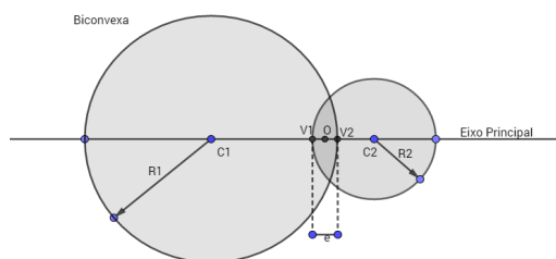
Figura 2: Lente Biconvexa
