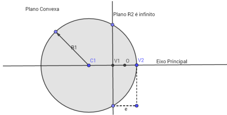
Figura 13 - Raio de curvatura e centro óptico de uma lente plano convexa.
