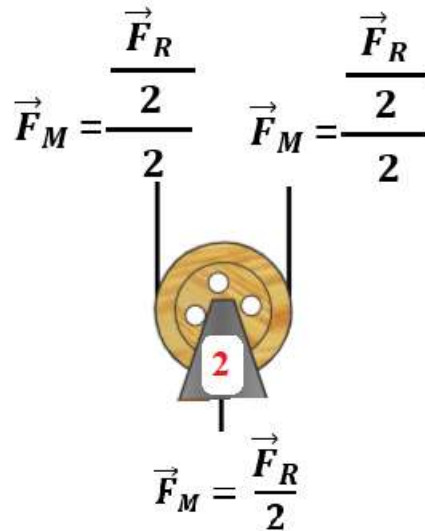
Figura 88 - Divisão das forças na polia 2 da associação de polias.
