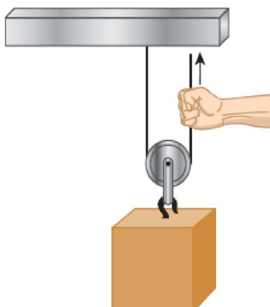
Figura 81 - Polia móvel.
