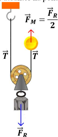
Figura 82 - Forças atuantes na polia móvel paralelas.
