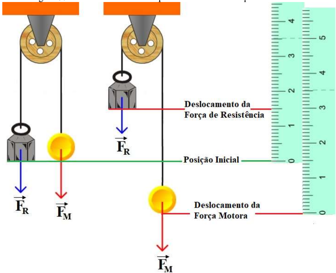
Figura 80 – Deslocamento entre o ponto final e inicial da polia fixa
