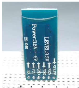
Figura 20 - Módulo bluetooth pinado na protoboard.
