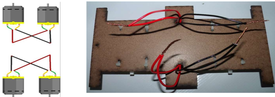
Figura 12 - União dos fios de mesma cor.
