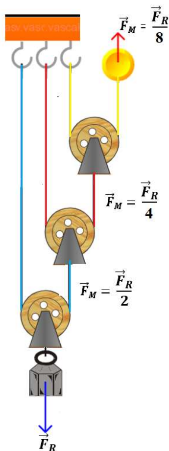
Figura 90 - Forças atuantes em cada polia dos sistemas de polias móveis
