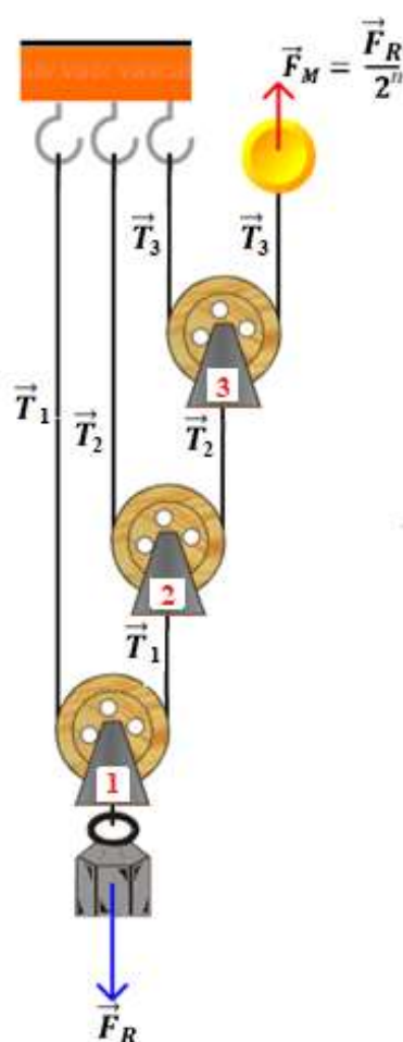
Figura 87 - Sistema de polias móveis.
