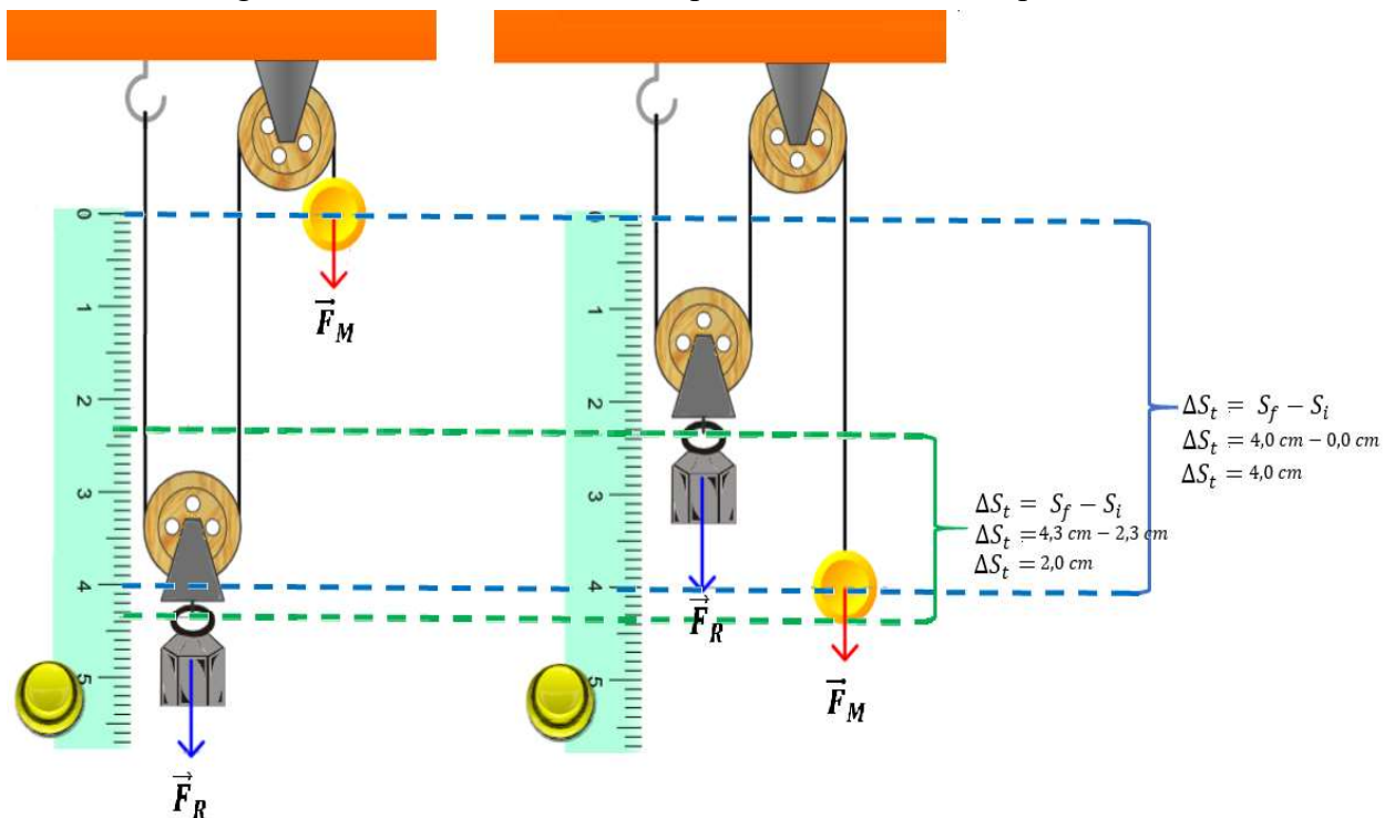
Figura 84 - Deslocamento entre o ponto inicial e final na polia móvel.
