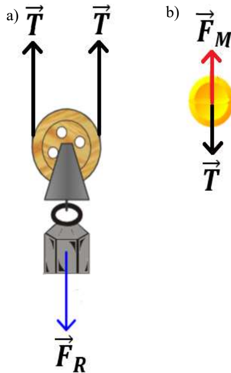
Figura 83 - Diagrama de corpo livre polia móvel
