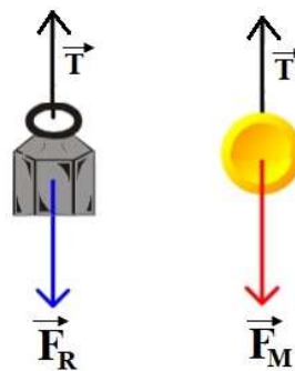
Figura 79 - Diagrama de corpo livre de uma polia fixa
