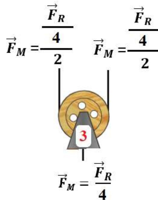
Figura 89 - Divisão de forças na polia 3 da associação de polias
