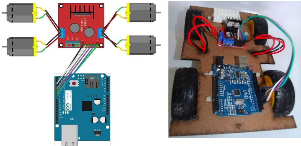
Figura 19 - Visão geral das conexões da placa Arduino e da ponte H.
