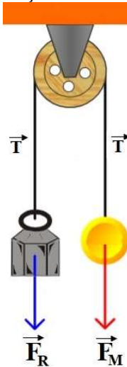
Figura 78 - Forças atuantes na polia fixa.
