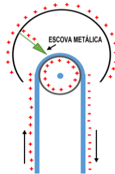
Figura 69: Escova metálica superior drenando cargas para a cúpula de descarga do GVDG.
