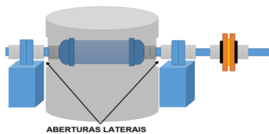
Figura 57. Eixo colocado por dentro das aberturas laterais da coluna de apoio.
