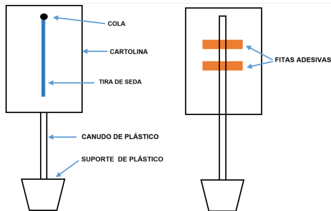
Figura 15: À esquerda a parte da frente do eletroscópio, e à direita a parte de trás.
