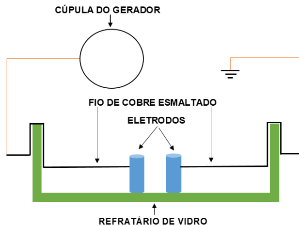
Figura 80: Esquema da montagem dos eletrodos e das ligações elétricas.
