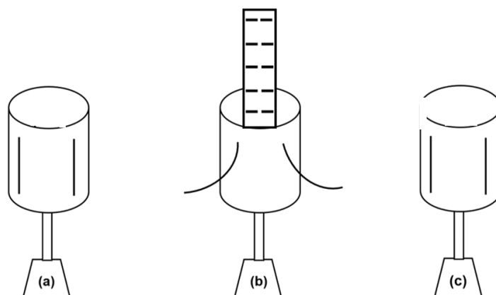
Figura 23: Em (a), a casca cilíndrica encontra-se neutra. Ao introduzir a régua eletrizada no interior da casca, as tirinhas se levantam. Em (c), ao retirar a régua do interior do cilindro, as tirinhas se abaixam.
