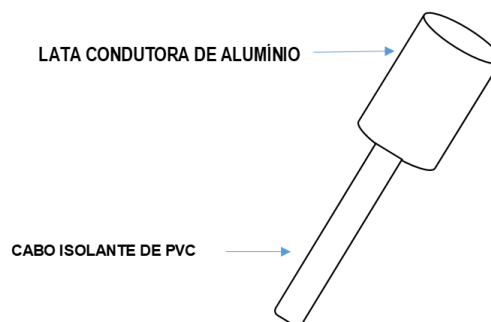
Figura 76: Centelhador feito de lata de alumínio e um pedaço de cano de PVC.
