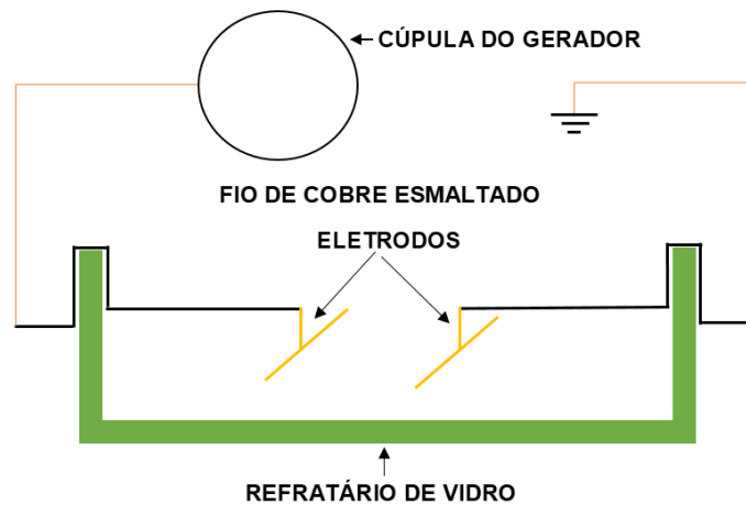
Figura 86: Eletrodos planos dispostos paralelamente.
