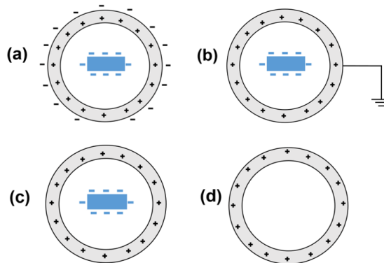
Figura 25: Vista de cima do cilindro. (a) A casca encontra-se com as cargas polarizadas devido à presença da régua eletrizada; (b) A casca é aterrada; (c) Desfaz-se o aterramento na presença da régua eletrizada; (d) Retira-se a régua.
