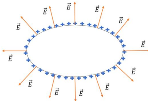
Figura 73: O campo elétrico é perpendicular à superfície do condutor em equilíbrio eletrostático.
