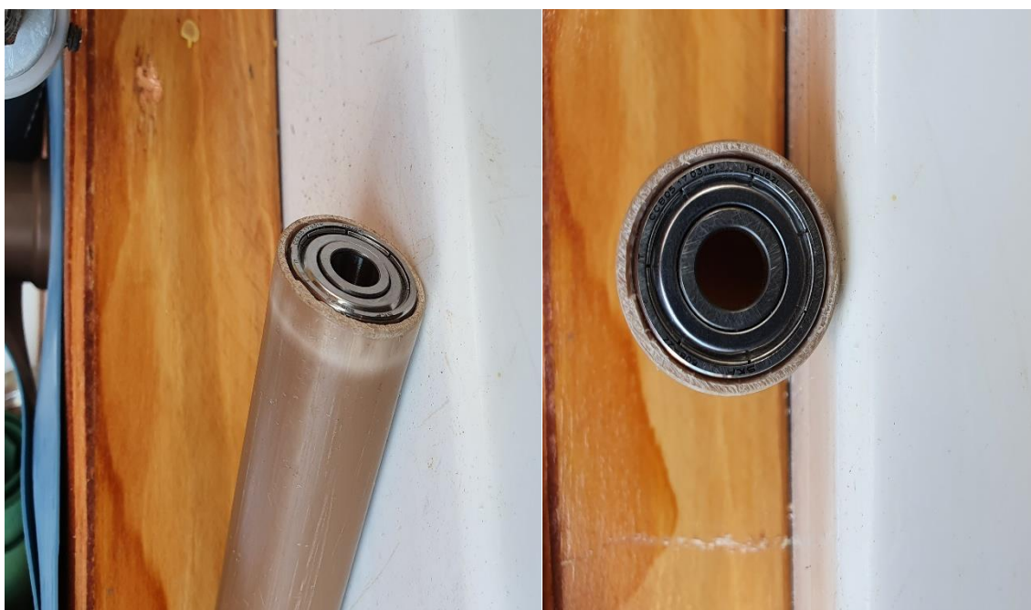
Figura 50: Rolamento de skate encaixado no cano de PVC usado no rolete superior.
