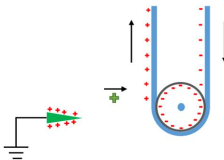
Figura 68: Íons positivos indo em direção à correia por meio do plasma condutor.
