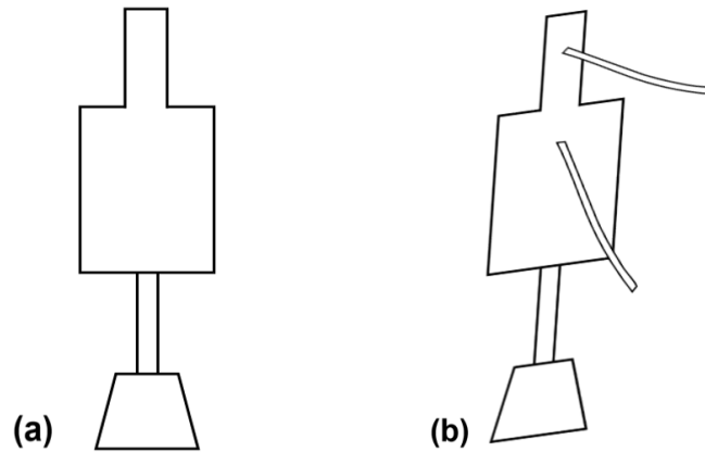
Figura 29: (a) Esquema do eletroscópio; (b) Após ser eletrizado, verifica-se que a tirinha que está na região da ponta se levanta mais, evidenciando que a concentração de cargas nessa região é maior.
