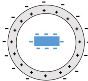
Figura 24: Vista de cima da casca cilíndrica. No centro, em azul, a régua eletrizada negativamente. Ao redor, em preto, a casca cilíndrica com suas cargas elétricas polarizadas.
