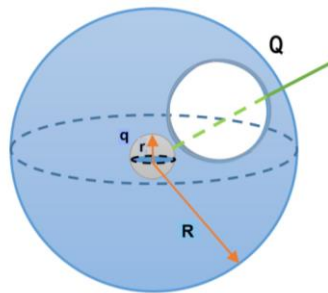
Figura 75: Esfera eletrizada q dentro da casca esférica que representa a cúpula de descarga do GVDG. A esfera eletrizada por sua vez, representa a porção eletrizada da correia transportadora de cargas.
