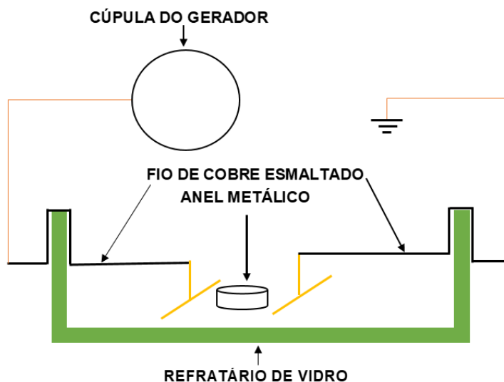
Figura 89: Esquema da montagem com anel metálico.
