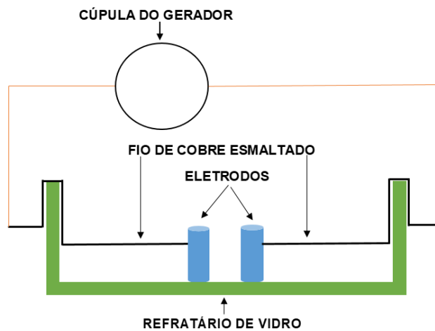
Figura 83: Esquema de montagem para eletrodos com cargas de mesmo sinal.
