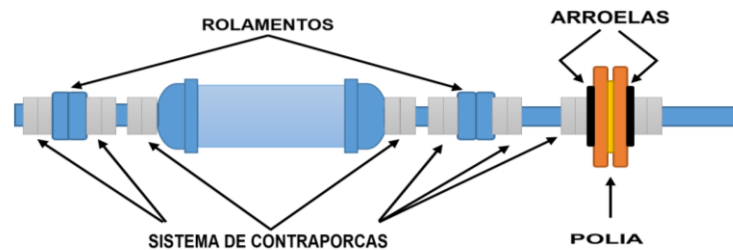
Figura 54: Eixo com polia acoplada.
