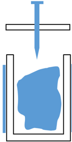
Figura 34: Esquema de montagem do capacitor cilíndrico. Em destaque, os materiais condutores na cor azul (palha de aço dentro do pote, prego e papel alumínio no lado externo do pote de plástico (dielétrico)).
