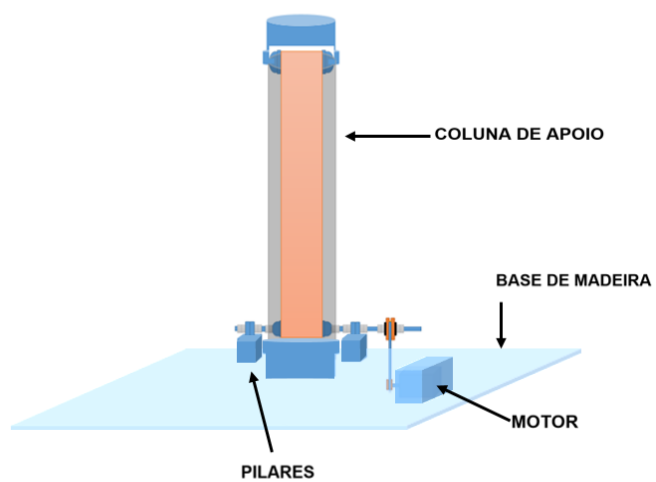
Figura 59: Esquema do GVDG montado.
