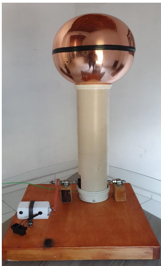
Figura 60: GVDG construído pelo autor.
