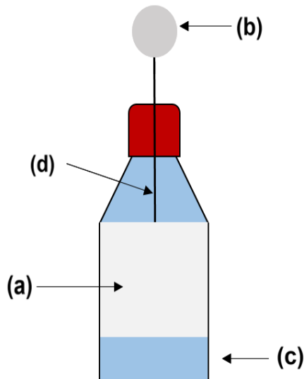
Figura 36: Esquema da garrafa de Leyden. (a) Fita de alumínio; (b) bola de papel alumínio; (c) água; (d) arame.
