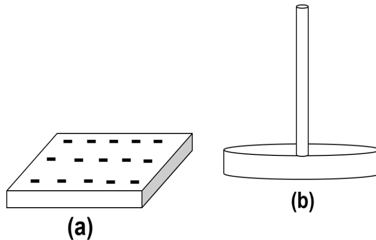
Figura 32: Em (a), a base isolante do eletróforo eletrizada; em (b), o coletor de cargas constituído pelo disco em alumínio com um pedaço de cano de PVC no seu centro.
