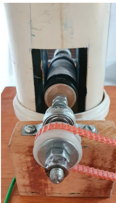
Figura 58: Eixo inferior alinhado com a abertura lateral da coluna de apoio (GVDG construído pelo autor)
