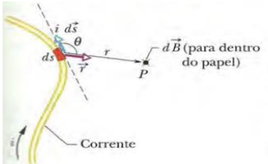
Figura 9 - Campo magnético produzido no ponto P pela carga presente no seguimento do fio.
