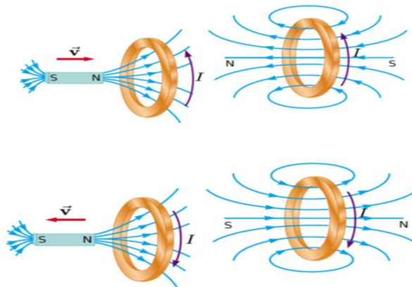
Figura 11 - Sentido da corrente e do campo magnético induzido, ao aproximar e afastar o ímã de uma espira.
