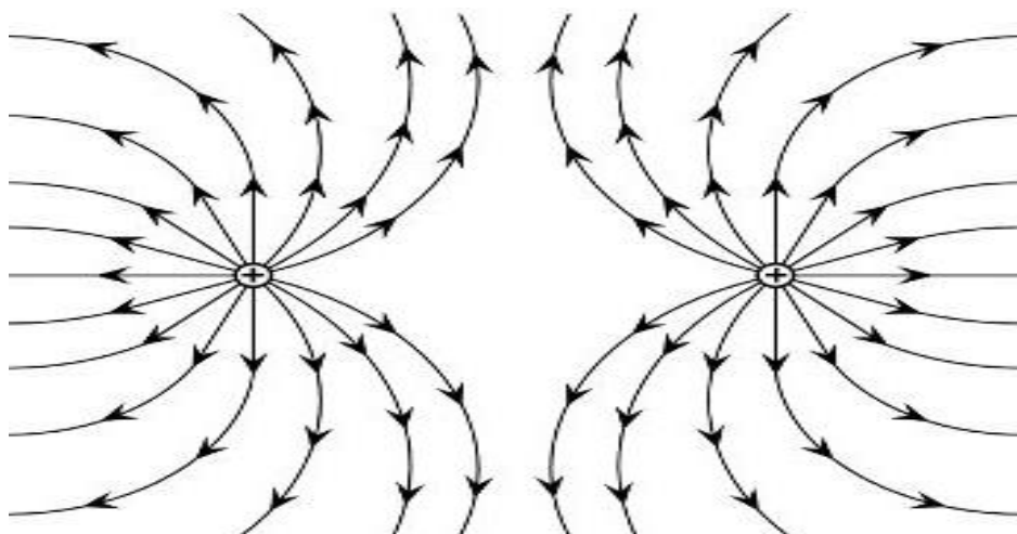
Figura 84: Configuração das linhas de força para dois eletrodos com cargas de mesmo sinal.
