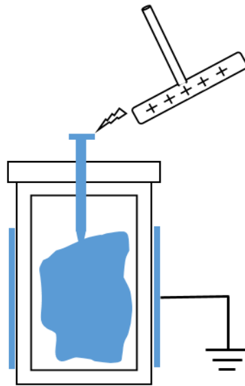
Figura 35: Capacitor sendo carregado pelo coletor de cargas do eletróforo. Mesmo sem o contato, as cargas são transferidas através do ar ionizado. Fonte:
