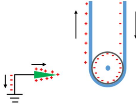
Figura 67: Polarização de cargas na escova metálica inferior.
