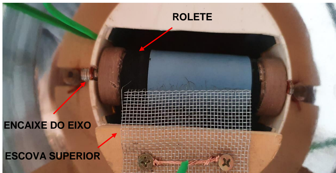
Figura 47: Rolete superior encaixado no cap superior.
