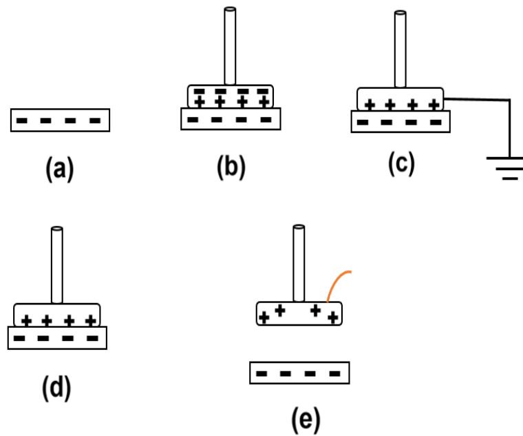
Figura 33: Processo de eletrização do coletor de cargas do eletróforo.
