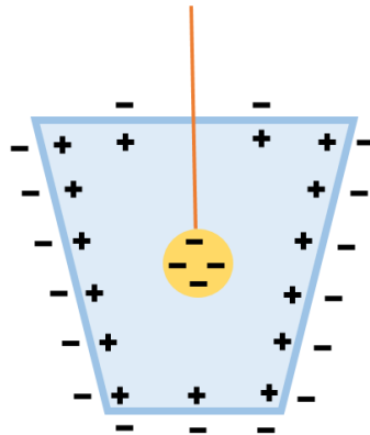
Figura 74: Separação das cargas elétricas do balde provocada pela presença da esfera eletrizada.
