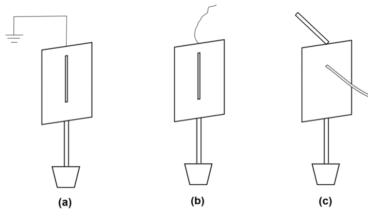
Figura 17: Tocando o eletroscópio carregado com diferentes tipos de materiais.
