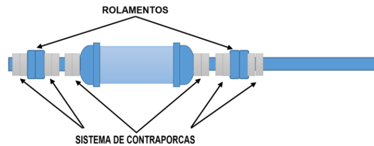
Figura 53: Eixo com os rolamentos colocados.
