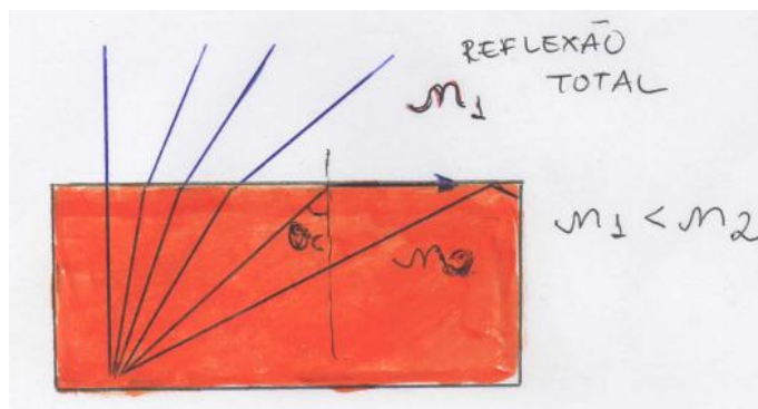
FIGURA 7: REFLEXÃO TOTAL DA LUZ E ÂNGULO CRÍTICO.
