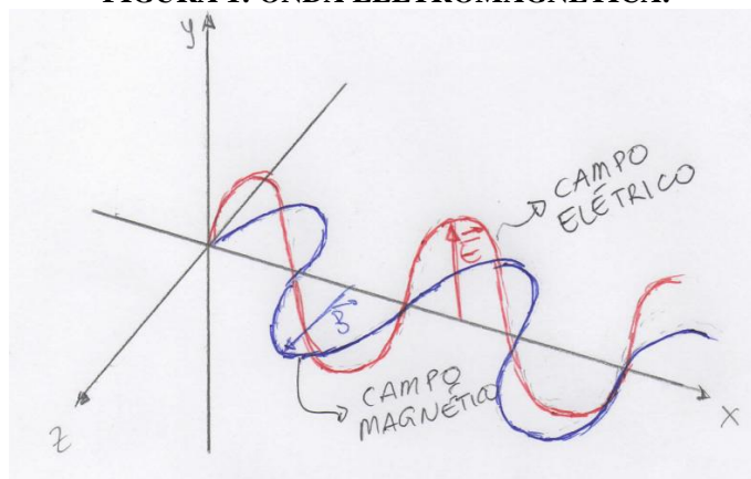
FIGURA 1: ONDA ELETROMAGNÉTICA.
