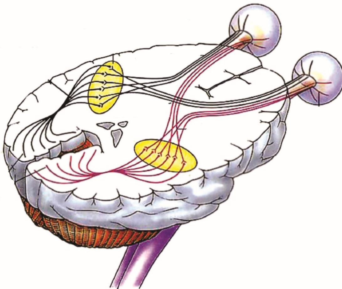
FIGURA 81 - SISTEMA VISUAL
