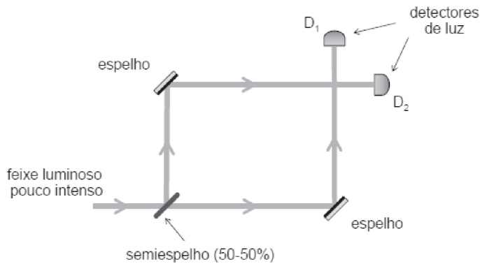
Figura 7.1 – Quando o feixe é dividido pelo semiespelho, os dois detectores podem clicar, de forma aleatória.
