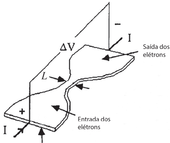
Figura 4.2 – Esquema da constrição de um gás de elétrons bidimensional para produzir um canal unidimensional de largura L ou fio quântico. Elétrons fluem de um terminal a outro devido ao potencial \Delta V .
