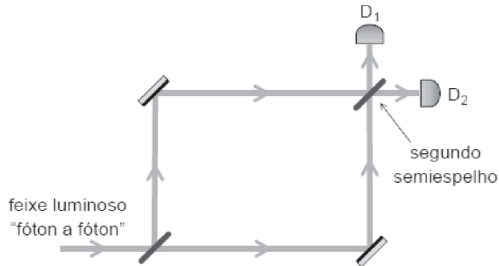
Figura 7.2 – Quando os feixes parciais são recombinados, existe interferência e apenas um dos detectores irá clicar.
