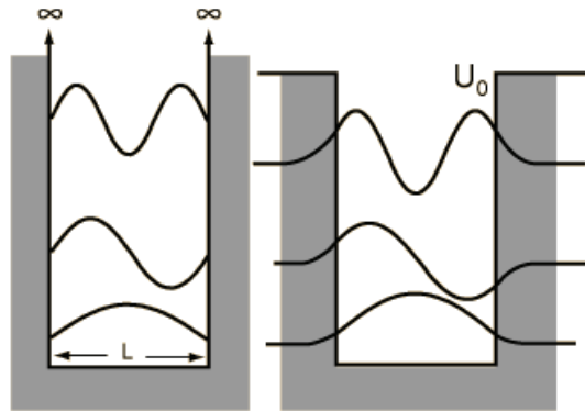
Figura 3.1 – Comparação entre o poço infinito e um poço finito. No segundo caso, as funções de onda estacionárias decaem exponencialmente a zero fora do poço.
