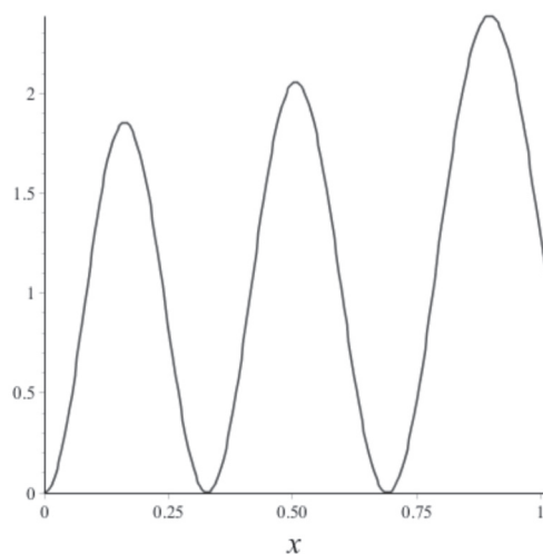
Figura 6.1 – Função de onda da Eq. (6.10) para a = 50 e \epsilon = 100 .
