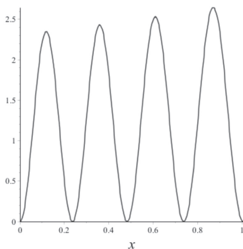
Figura 6.2 – Função de onda da Eq. (6.10) para \alpha = 50 e \epsilon = 182 .
