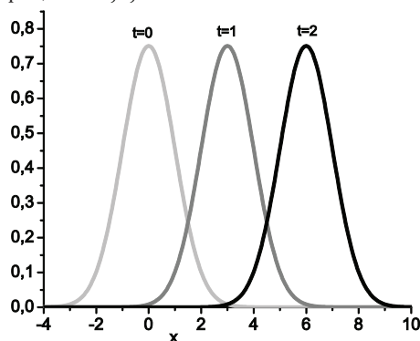
Figura 1.2 – Evolução de uma densidade Gaussiana, inicialmente centrada na origem, para uma partícula livre com velocidade v=3 . Note como a função se propaga sem alterar sua forma.
