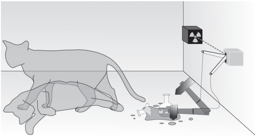
Figura 8-1 – Ilustração da experiência de pensamento de Schrödinger. Fonte: Wikipedia.
